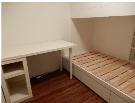
1階ベッド側、既存デスクをカットし再利用
